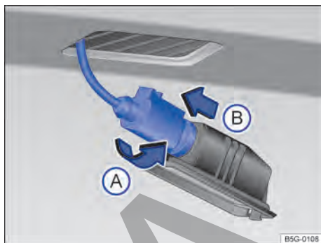
Fig. 132 Luz de la placa de licencia: desinstalar el portalámparas.
