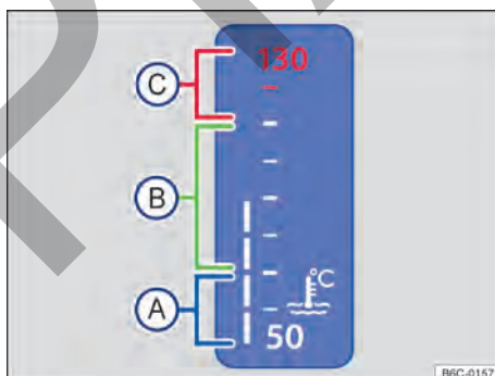
Fig. 17 Indicador de temperatura del líquido de refrigeración del motor en instrumento combinado digital: (A) zona fría; (B) zona normal; (C) zona de alerta.
