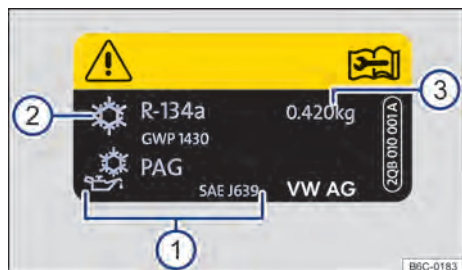
Fig. 169 Información del aire acondicionado.
