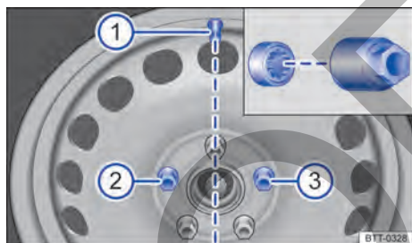
Fig. 161 Cambio de rueda: válvula del neumático ① y posición de montaje del tornillo de la rueda antirrobo ② o ③.
