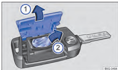
Fig. 50 Llave del vehículo: sustituir la pila.
