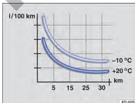
Fig. 86 Consumo de combustible en l/100 km en 2 temperaturas ambiente distintas.
