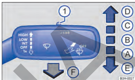
Fig. 74 A la derecha de la columna de dirección: comandar los limpiaparabrisas.
