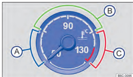
Fig. 16 Indicador de temperatura del líquido refrigerante del motor en el instrumentos combinado analógico (variante 2) : (A) zona fría; (B) zona normal; (C) zona de alerta.
