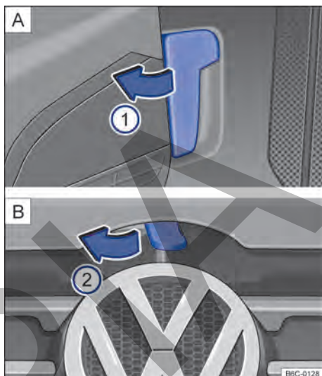
Fig. 141 [A] Palanca de desbloqueo de la tapa del compartimento del motor en la zona reposapiés del conductor. [B] Palanca de desbloqueo en la parte interior de la tapa del compartimento del motor.
