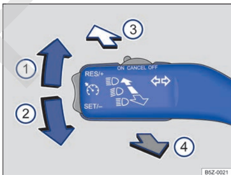
Fig. 77 Palanca de los indicadores de dirección y del faro alto en la posición básica.
