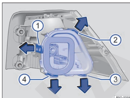
Fig. 179 Grupo óptico trasero en la carrocería: desmontaje del portalámparas. ① a ④ pestañas de bloqueo.
