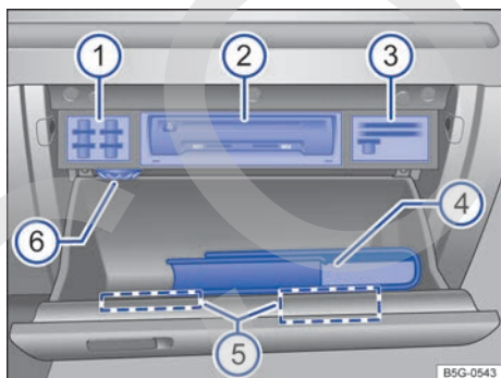
Fig. 142 Guantera abierta.
