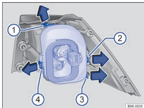
Fig. 177 Grupo óptico trasero en la carrocería: desmontaje del portalámparas. ① a ④ pestañas de bloqueo.
