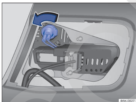
Fig. 175 En el portón del maletero: extraer el portalámparas.
