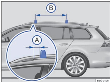
Fig. 162 Barra longitudinal del techo: fijación de las barras transversales.
