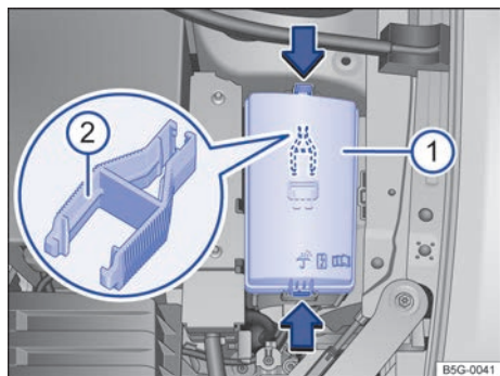
Fig. 183 En el vano motor: cubierta ① de la caja de fusibles con pinzas de plástico ②.
