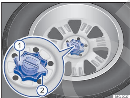
Fig. 206 En el maletero: ruedecilla para fijar la rueda de repuesto.
