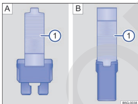
Fig. 185 Extraer o colocar el fusible con las pinzas de plástico: A Fusible enchufable plano. B Fusible tipo bloque.
