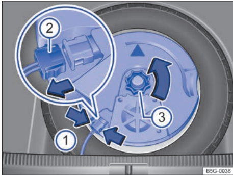
Fig. 218 En el maletero: desmontar el subwoofer (variante 1).
