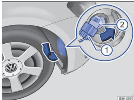
Fig. 169 En el guardabarros delantero derecho: cambio de lámpara en el faro.
