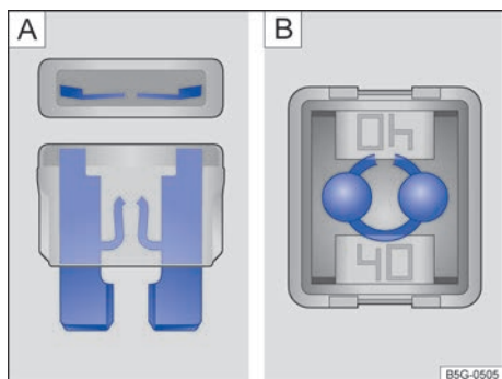
Fig. 184 Fusible fundido: A Fusible enchufable plano. B Fusible tipo bloque.
