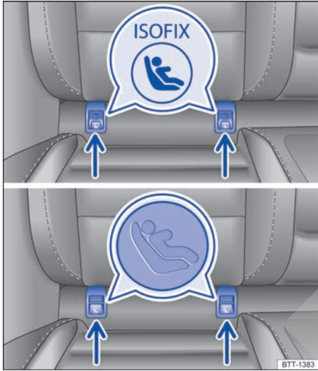
Fig. 26 En el asiento del vehículo: tipos de señalización de los puntos de anclaje ISOFIX para los asientos para niños.
