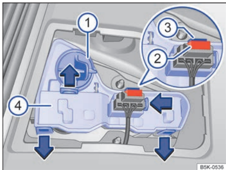
Fig. 171 En el portón del maletero: extraer el portalámparas.
