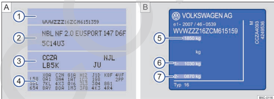
Fig. 223 A Portadatos del vehículo: en la figura, por ejemplo, con letras distintivas del motor CCZA 3. B) Placa de modelo.
