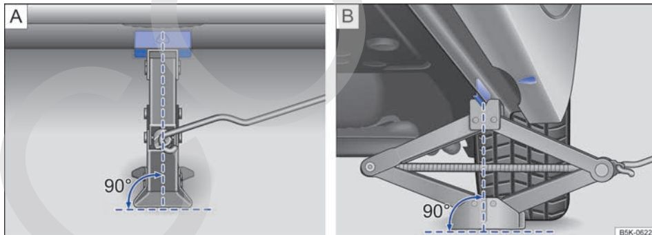
Fig. 217 Gato colocado en el lado izquierdo del vehículo, en la zona trasera.
