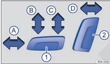
Fig. 76 Mandos en el asiento delantero izquierdo: ajuste longitudinal del asiento, ajuste de la altura y de la inclinación de la banqueta, y ajuste del respaldo.
