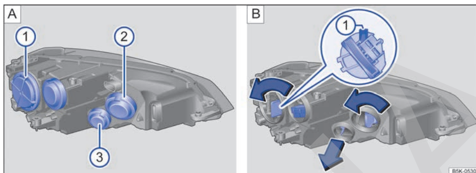
Fig. 167 En el vano motor: tapas del faro izquierdo. ① luz de cruce, ② luz de carretera, luz de posición y luz diurna, ③ intermitente.
