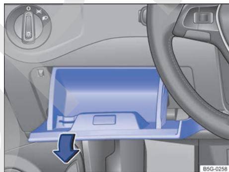
Fig. 182 En el lado izquierdo, junto al volante: tapa de la caja de fusibles del tablero de instrumentos. ▶
