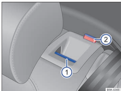
Fig. 78 En el respaldo del asiento trasero: tecla de desbloqueo ①; marca roja ②.
