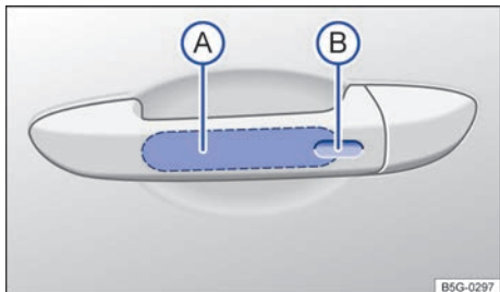
Fig. 55 Sistema de cierre y arranque sin llave Keyless Access: superficie sensora (A) de desbloqueo en el lado interior de la manilla de la puerta y superficie sensora (B) de bloqueo en el lado exterior de la manilla.
