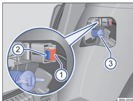
Fig. 176 Lateral del maletero: desmontaje del grupo óptico trasero. ▶
