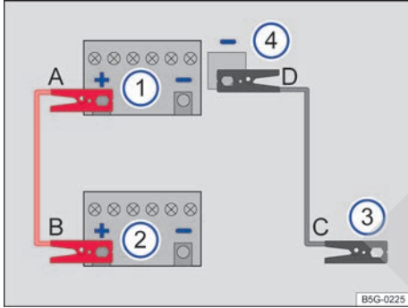
Fig. 187 Esquema para conectar los cables de arranque en el caso del vehículo que suministra la co- rriente.
