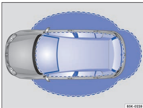
Fig. 54 Sistema de cierre y arranque sin llave Keyless Access: zonas de proximidad.
