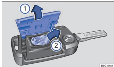
Fig. 51 Llave del vehículo: cambiar la pila de botón.
