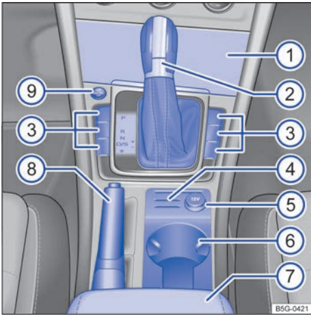
Fig. 37 Cuadro general de la parte inferior de la consola central.
