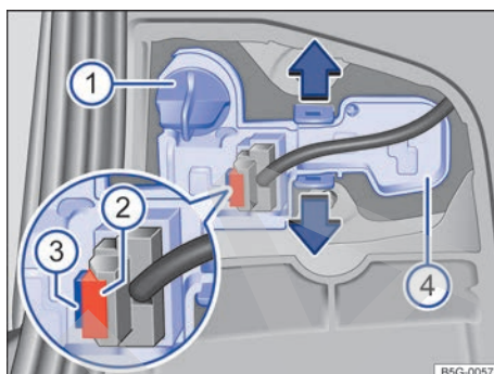
Fig. 173 En el portón del maletero: extraer el portalámparas.
