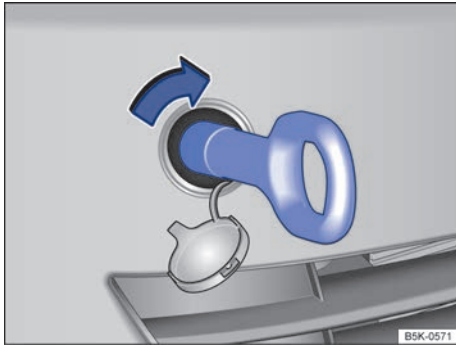
Fig. 189 En el lado derecho del paragolpes delantero: enrosca la argolla de remolque.
