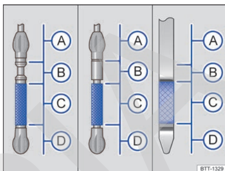
Fig. 196 Varilla de medición con marcas del nivel del aceite del motor.
