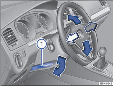
Fig. 73 Debajo del volante, en el guarnecido de la columna de dirección: palanca para el ajuste manual de la posición del volante.
