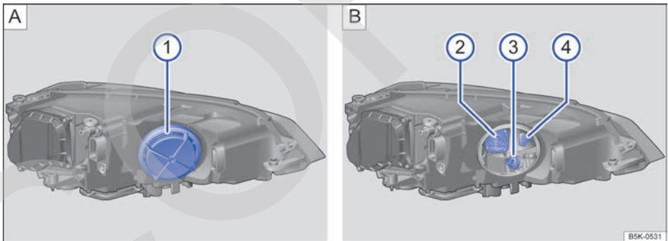
Fig. 168 En el vano motor: ① tapa en el faro izquierdo, ② luz de curva estática, ③ intermitente, ④ luz de posición y luz diurna independiente.
