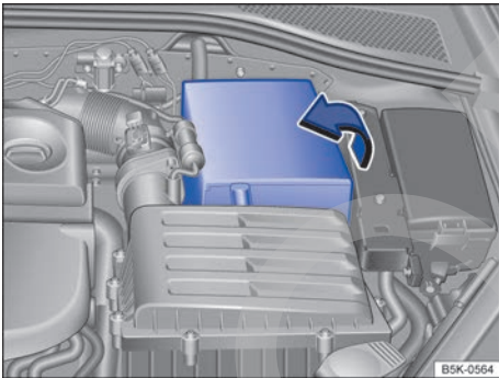
Fig. 200 En el vano motor: levantar la cubierta guardapolvo de la batería de 12 voltios.
