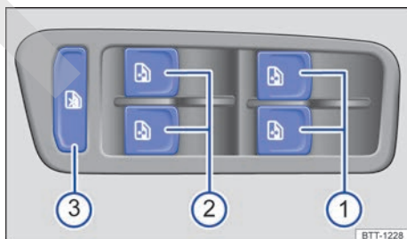
Fig. 63 En la puerta del conductor: teclas de los elevalunas delanteros y traseros.
