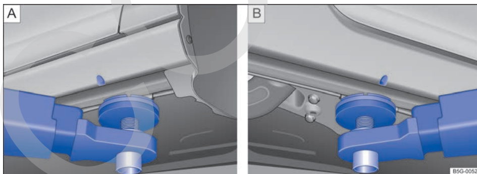
Fig. 221 A Punto de apoyo en la parte delantera y B punto de apoyo en la parte trasera para elevar el vehículo con la plataforma elevadora o el gato (variante 1).
