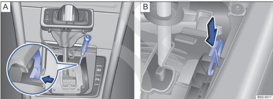
Fig. 72 Debajo de la cubierta de la corredera de la palanca selectora: desbloqueo de emergencia del bloqueo de la palanca selectora (variante A y variante B).
