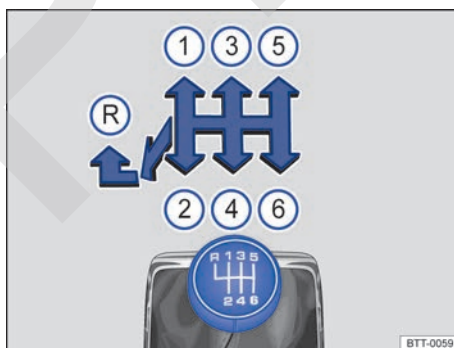
Fig. 116 Esquema de un cambio manual de 6 marchas.
