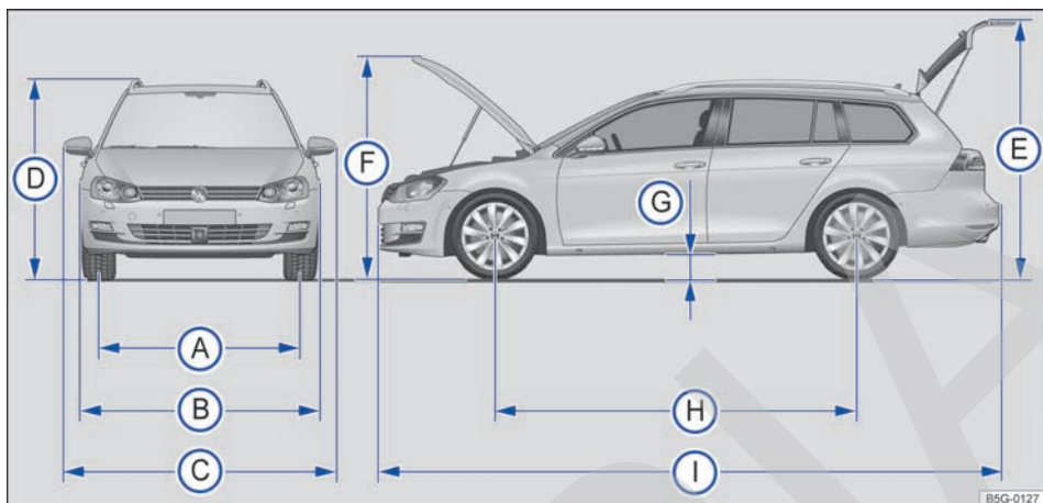
Fig. 225 Dimensiones.
