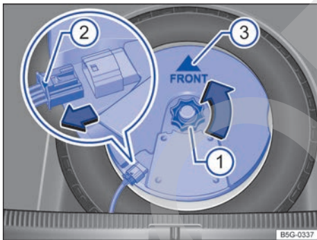
Fig. 219 En el maletero: desmontar el subwoofer (variante 2).
