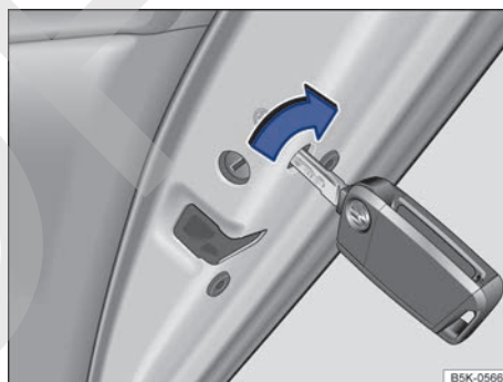
Fig. 68 En el frontal de la puerta trasera derecha: bloqueo de emergencia del vehículo con la llave del vehículo.
