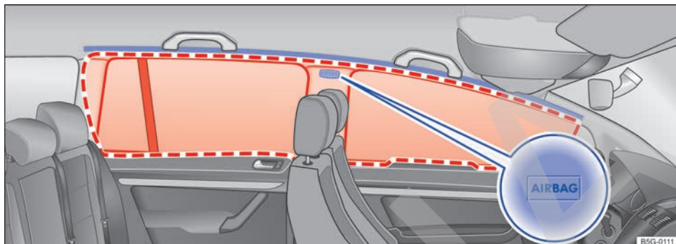
Fig. 20 En el lado izquierdo del vehículo: ubicación y zona de despliegue del airbag para la cabeza.
