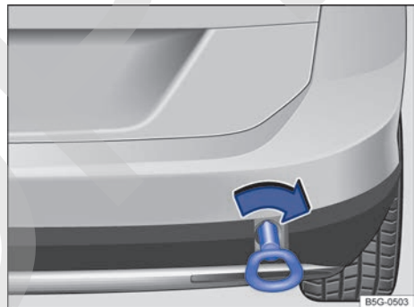
Fig. 191 En el lado derecho del paragolpes trasero: enrosca la argolla de remolque.
