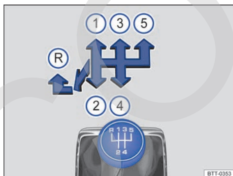
Fig. 115 Esquema de un cambio manual de 5 marchas.
