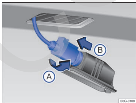
Fig. 181 Luz de matrícula: desmontaje del portalámparas.
