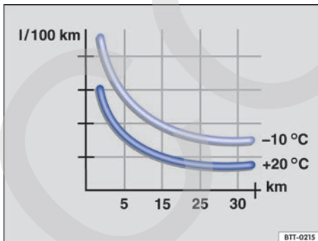
Fig. 109 Consumo de combustible en l/100 km a dos temperaturas ambiente diferentes.
