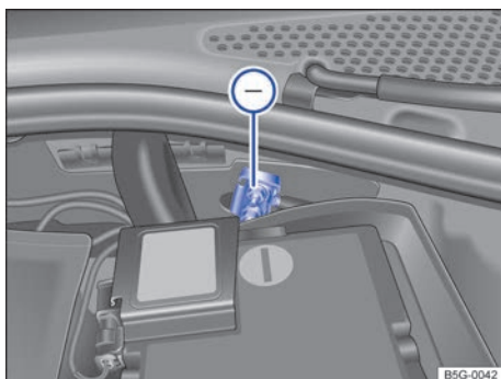
Fig. 186 En el vano motor: toma para la ayuda de arranque (terminal de masa) (-).
