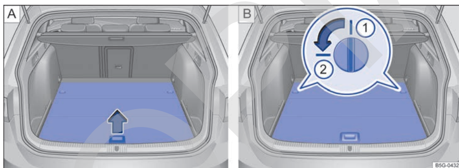
Fig. 160 En el maletero: A Levantar el piso del maletero. B Posición ①: bloqueo del piso del maletero cerrado, posición ②: bloqueo abierto.
