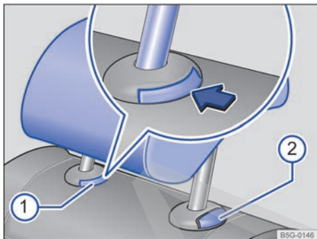
Fig. 83 Desmontaje de los apoyacabezas traseros.
