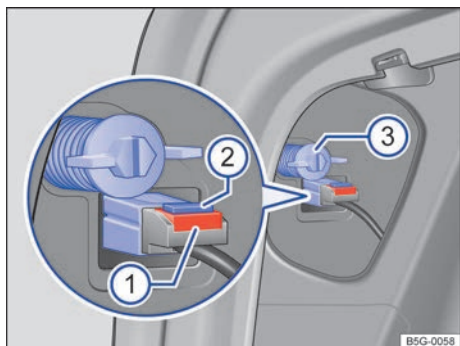
Fig. 178 Lateral del maletero: desmontaje del grupo óptico trasero.
