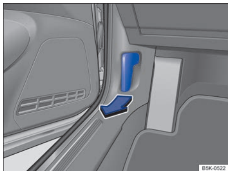
Fig. 192 En la zona reposapiés del lado del conductor: palanca de desbloqueo del capó del motor.
