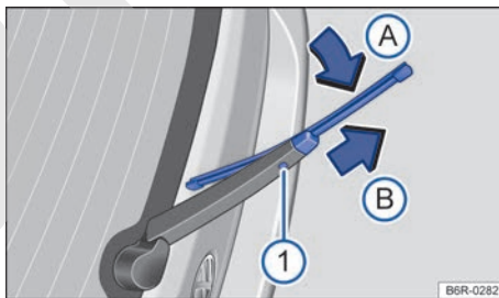
Fig. 94 Cambio de la escobilla limpiacristales de la luneta.
