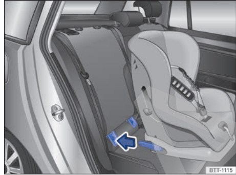
Fig. 27 Representación esquemática: montaje de un asiento para niños ISOFIX con conectores.
