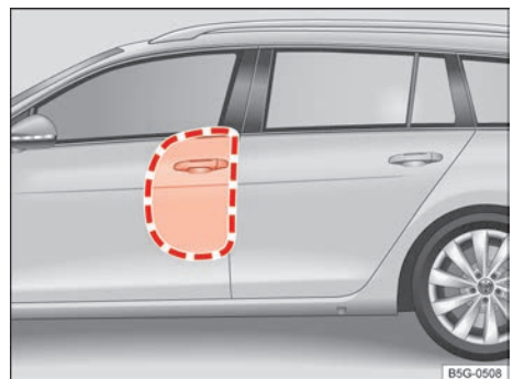
Fig. 18 En el lado izquierdo del vehículo: zonas de despliegue del airbag lateral. ▶
