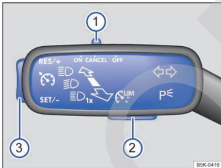
Fig. 121 En el lado izquierdo de la columna de dirección: mando y teclas para manejar el GRA.
