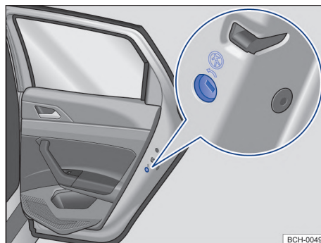
Fig. 48 En la puerta trasera (lado derecho): ubicación del seguro para niños.
