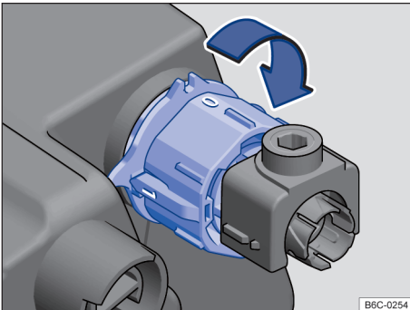
Fig. 74 En el compartimento del motor: conmutador de regulación del alcance de las luces.
