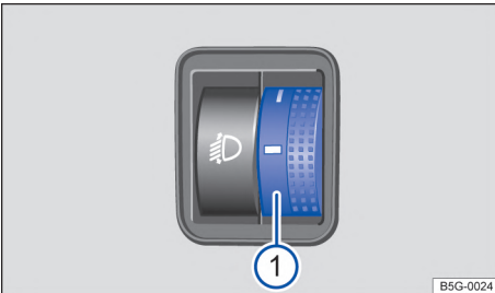
Fig. 73 Al lado del volante: regulador de alcance del faro ①.
