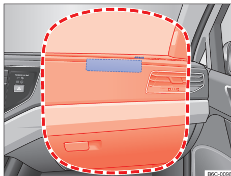
Fig. 38 Ubicación y radio de expansión del airbag frontal del acompañante.
