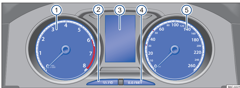
Fig. 10 instrumento combinado analógico.
