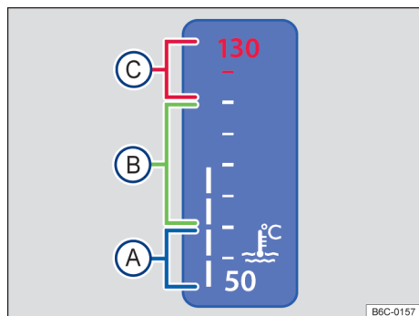
Fig. 15 Indicador de temperatura del líquido refrigerante del motor en el instrumento combinado digital (variante 1): (A) zona fría; (B) zona normal; (C) zona de alerta.
