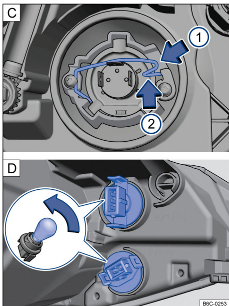
Fig. 166 En el compartimento del motor: cubierta de los intermitentes de las luces de carretera y del faro bajo.
