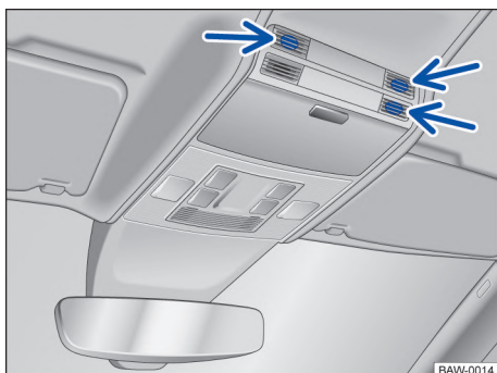
Fig. 60 En la consola del techo: sensores de vigilancia del habitáculo (flechas).
