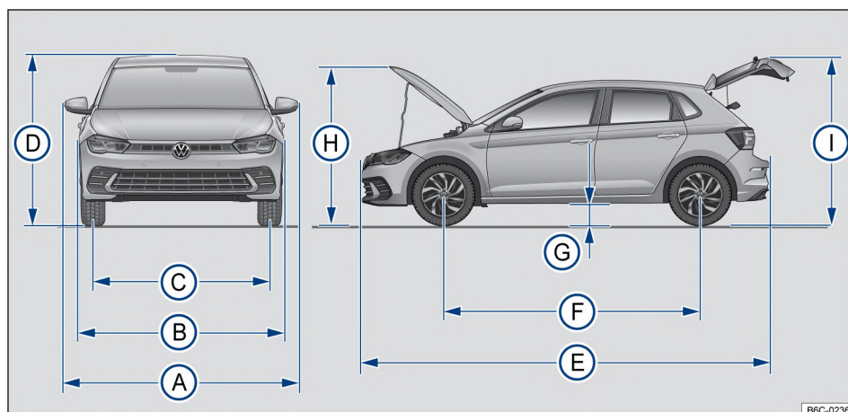
Fig. 208 Dimensiones.
