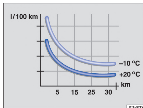
Fig. 88 Consumo de combustible en l/100 km en 2 temperaturas ambiente diferentes.
