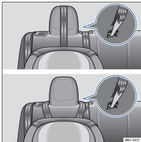
Fig. 46 En el respaldo del asiento trasero: A ) colocación de la banda del cinturón en el caso de apoyacabezas no ajustables con cinturón individual Top Tether, B ) colocación de la banda del cinturón en el caso de apoyacabezas no ajustables con cinturón Top Tether en forma de V.
